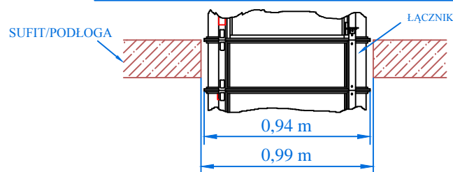
SKALA 2:1 (STANDARDOWY OTWÓR SUFIT/PODŁOGA)
